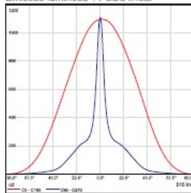
Emissão luminosa 1 / CDL linear
