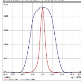
Emissão luminosa 1 / CDL linear
