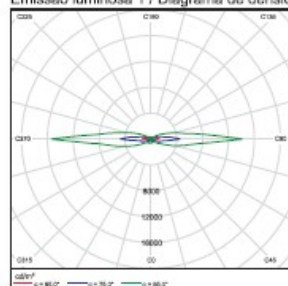
Emissão luminosa 1 / Diagrama de densidade de luminância
