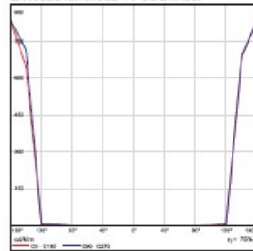
Emissão luminosa 1 / CDI, linear
