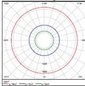
Emissão luminosa 1 / Diagrama de densidade de luminância
